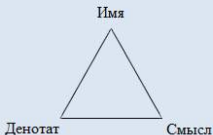
Рис.1. Семантический треугольник
