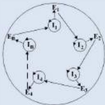
Рис.2. Структура гиперцикла.
